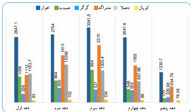
شکل ۲- تغییرات دبی بیک در ۵ دهه اخیر در ایستگاه‌های مشرف به کانون‌های گرد و غبار
