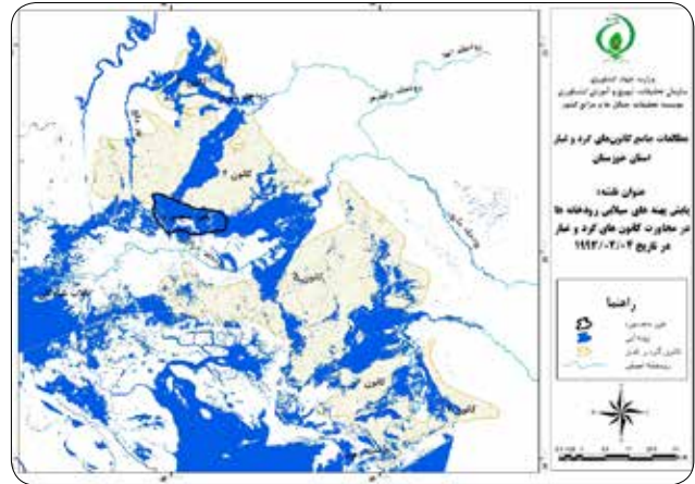
شکل ۳- پهنه‌های سیلابی در سیلاب به تاریخ ۱۹۹۲/۰۴/۰۲ (تاریخ معادل شمسی ۱۳۷۱/۱۱/۱۵)
