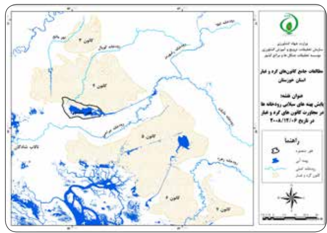
شکل ۵- پهنه‌های سیلابی در سیلاب به تاریخ ۲۰۰۸/۱۲/۰۶ (تاریخ معادل شمسی ۱۳۸۷/۰۹/۱۶)
