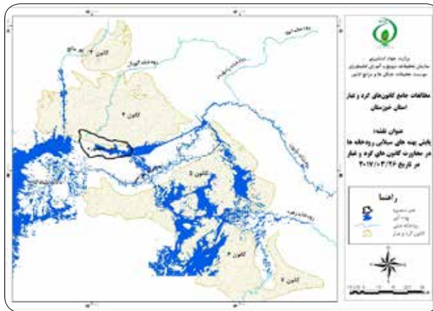
شکل ۶- پهنه‌های سیلابی در سیلاب به تاریخ ۲۰۱۷/۰۳/۲۶ (تاریخ معادل شمسی ۱۳۹۶/۰۱/۰۶)
